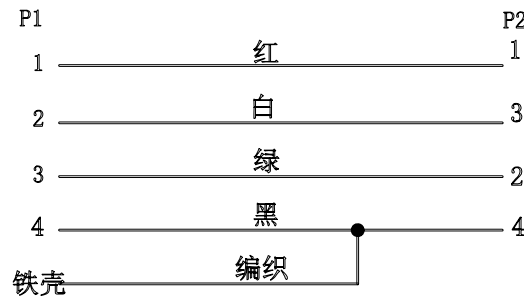
接点图
