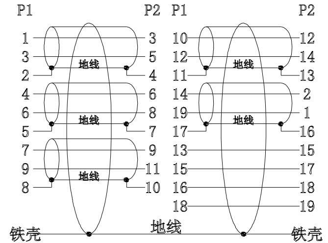
接点表
